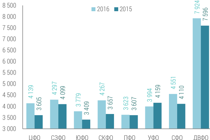
Средние цены приобретения цемента по округам РФ в январе-феврале 2016-2017 гг., руб./т с НДС и доставкой
