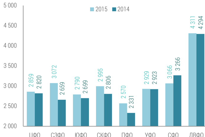
Средние цены производителей цемента по округам РФ в январе-июне 2014-2015 гг., руб./т без НДС и доставки
