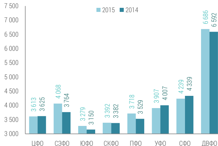
Средние цены приобретения цемента по округам РФ в январе-июне 2014-2015 гг., руб./т с НДС и доставкой
